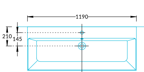
монтаж с раковиной GR.WB.120.1
