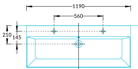
монтаж с раковиной GR.WB.120.2
