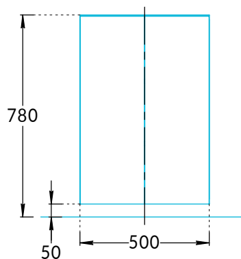
Монтаж со столешницей без выреза (KMCATp50MBt0, KMCATp50MMp0)
