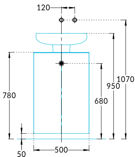
Монтаж с раковиной Safi (KMSFWb46GWb0, KMSFWb46MBIs0)
